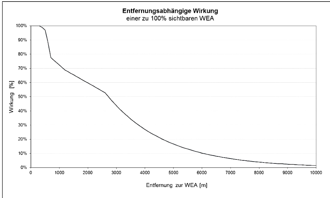
Abbildung 1: Bewertungsgraph Entfernung-Wahrnehmungsstärke nach Peters, Torkler, Brahms und Zeidler 10
