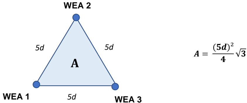
Abbildung 2: Anordnung von 3 Windenergieanlagen (WEA) im minimalen Abstand
